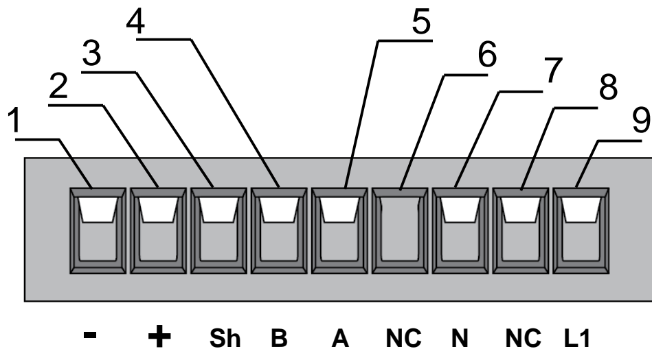
Рис. 2.3. Клеммный коннектор (а)
