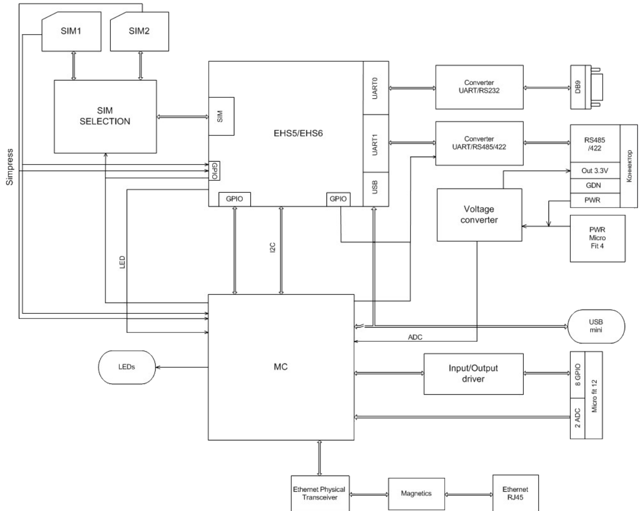
Рис. 3.1 Функциональная схема GSM-модема TU41
