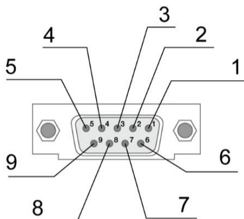
Рис. 2.4. Разъём DB9
