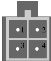
Рис. 2.6. Разъем питания (Microfit 4)
