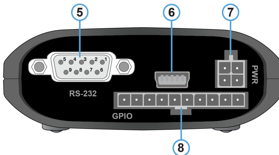
Рис. 2.2. Вид сзади
