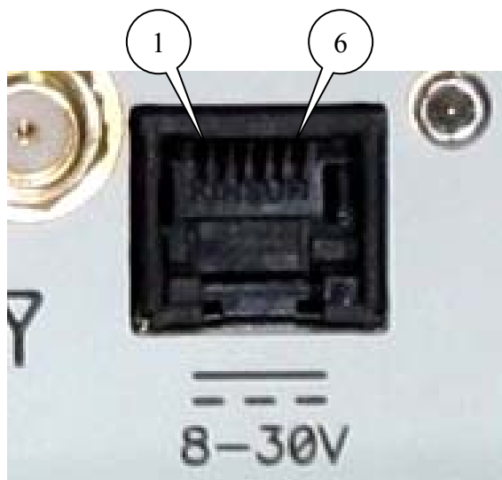
Рис.2.6.2 Разъём RJ11
